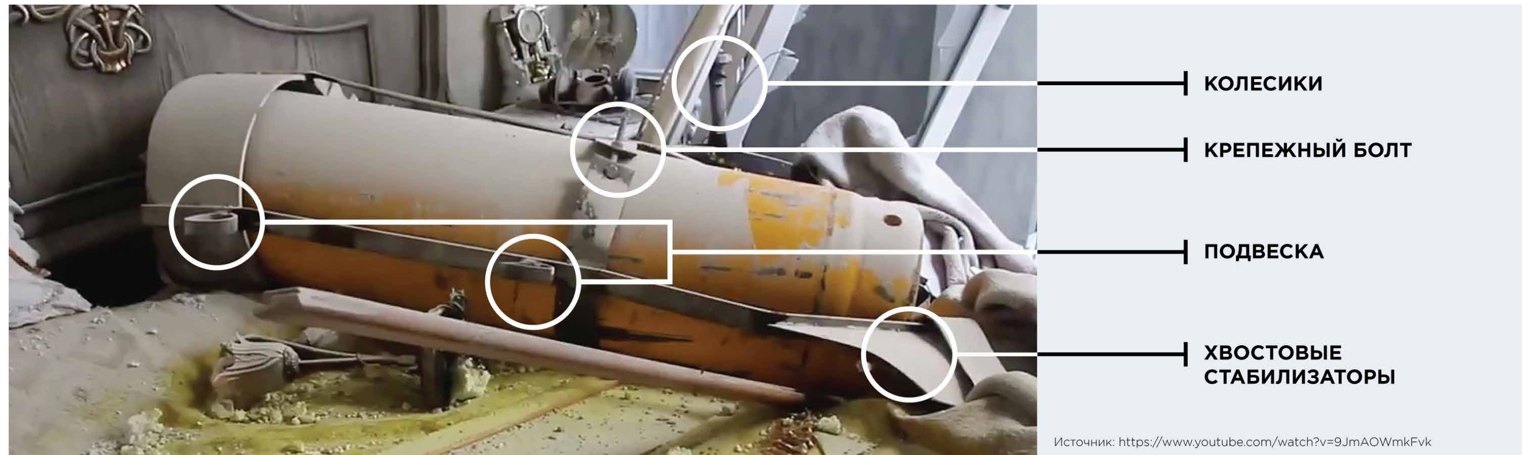
Обломки хлорного баллона с металлической внешней конструкцией, снятые на месте падения на балконе на видео, опубликованном 9 апреля 2018 г (Источник - Baladi-News Network, Youtube, 9 апреля 2018 г, https://www.youtube.com/watch?v=9JmAOwMkFvk )
