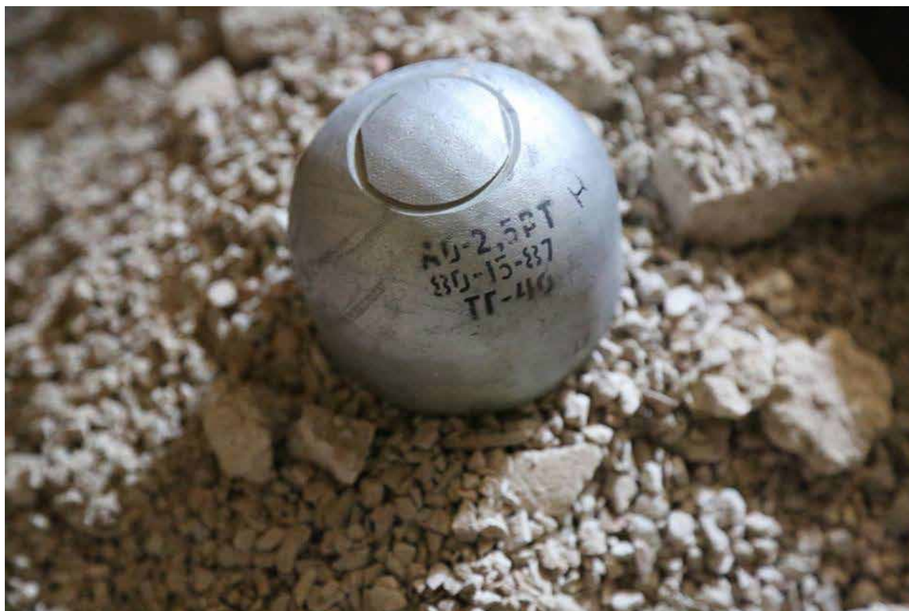
Обломки суббоеприпаса АО-2,5РТ, сфотографированные, как сообщается, в населенном пункте Сабка 11 марта 2018 г, на которых видны маркировки (Источник -Syrian Civil Defense - The White Helmets, Фейсбук, 11 марта 2018 г, https://www.facebook.com/SyriaCivilDef/photos/a.1712251465765921/2028943330763398/?type=3&theater ).
